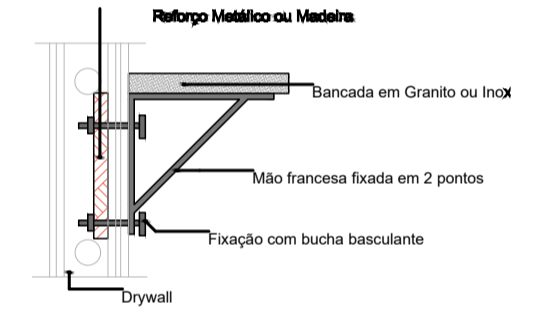
DETALHE 01: REFORÇO EM DRYWALL
